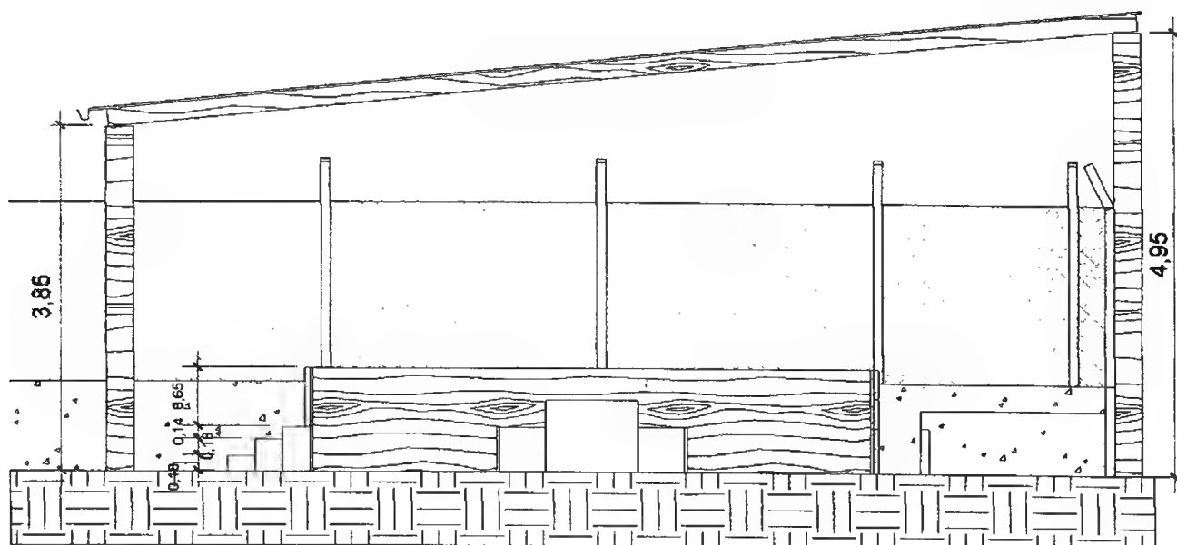
8 Corte AA 1:75
