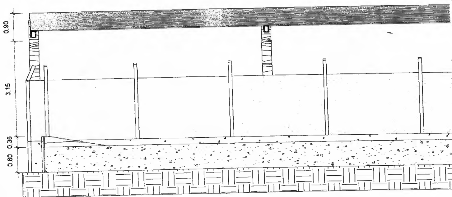
5 Corte BB 1:75
